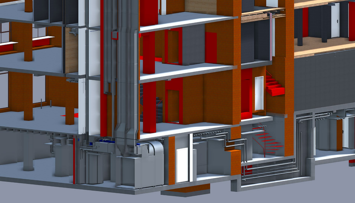
3D-Koordinationsmodell
